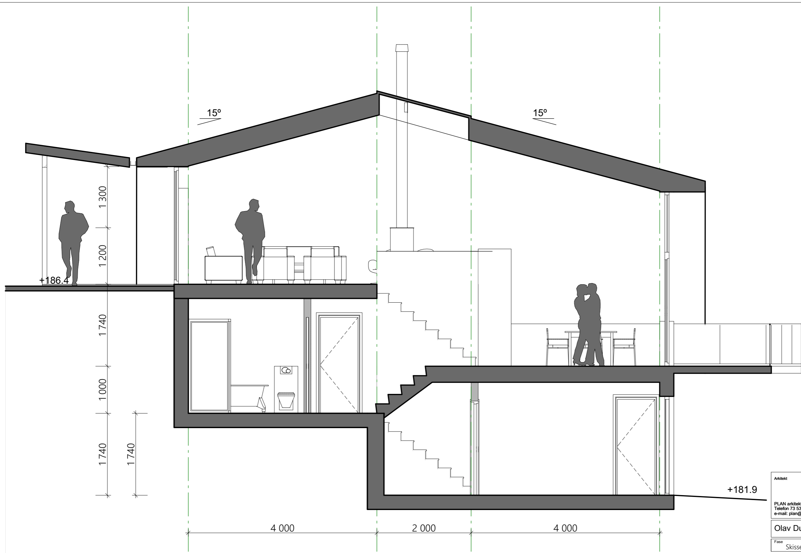
1:50 Snitt 2
